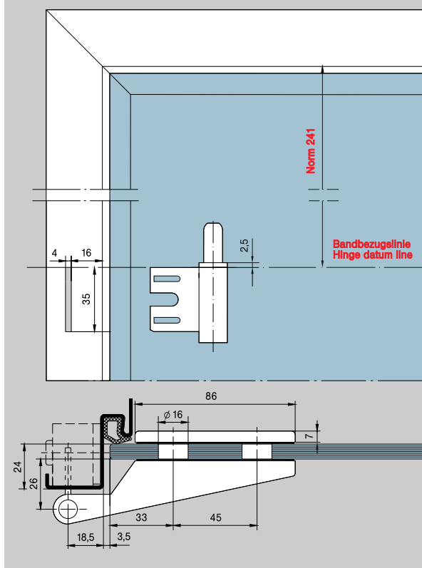
Aufschraub-Rahmenteil
